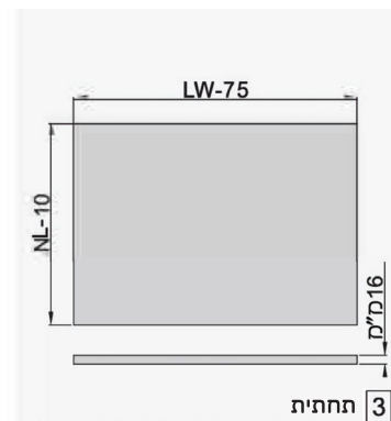
2 חזית
