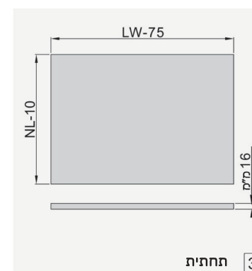
חזית 2
