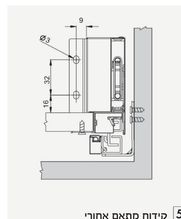
גב 4
